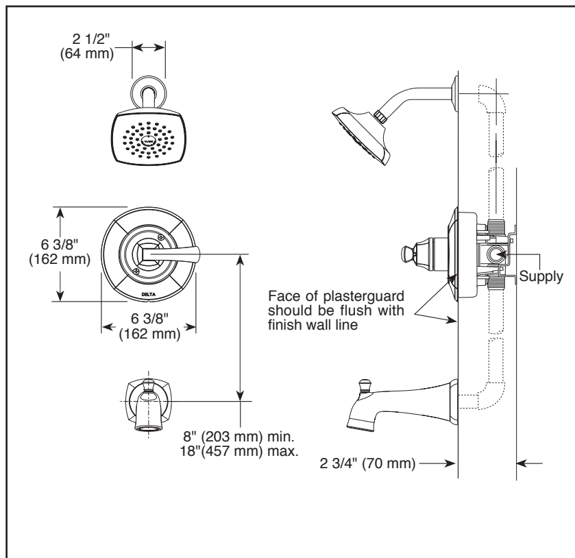
RP64862▲ (Pull-up Diverter)
